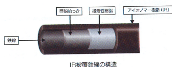
IR被覆鉄線の構造
